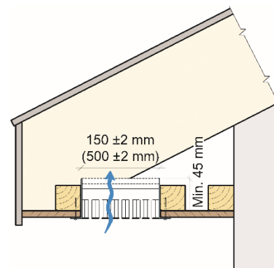
Fig. 2 Prinsipp for montering av Sealmaster lufteventil. For å oppnå en total brannmotstand på 30 minutter for raftet må omliggende konstruksjon også utføres med en tilsvarende brannmotstand.
