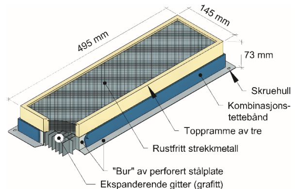
Fig. 1 Sealmaster brannhemmende lufteventil. Prinsipiell oppbygning. Brutto mål inkl. flens er 185x535x73 mm
